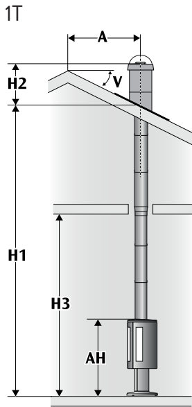
Halvisolert startør med overgang skjult i bjelkelag.
