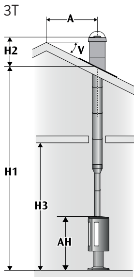
Uisolert startør.
