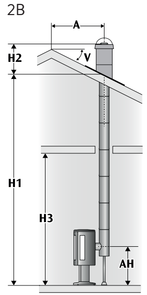
Bakmontert direkte bak ildsted. Helisolert pipe.
