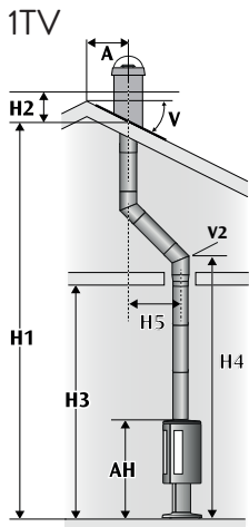
Toppmontering med halvisolert startør og senterforskyvning.
