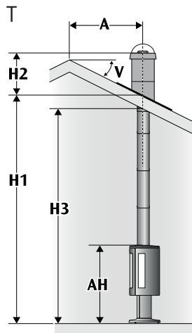
Toppmontert halvisolert
