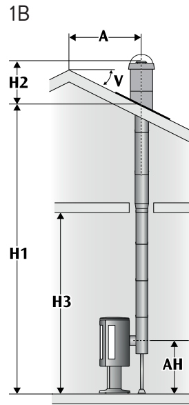
Bakmontering direkte bak ildsted. Halvisolert startør med overgang skjult i bjelkelag.
