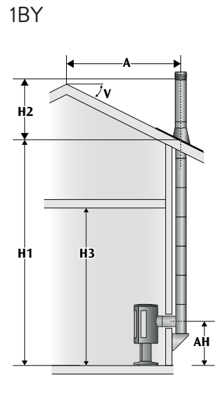
Bakmontering gjennom yttervegg.
