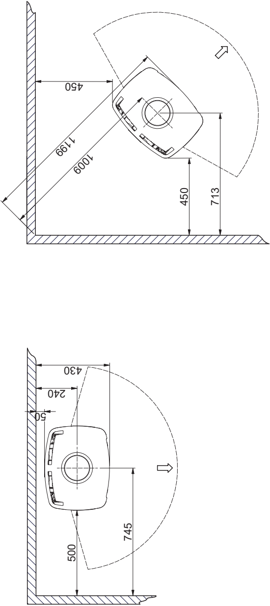
Minimumsavstand til brennbart materiale (med sideglass)
