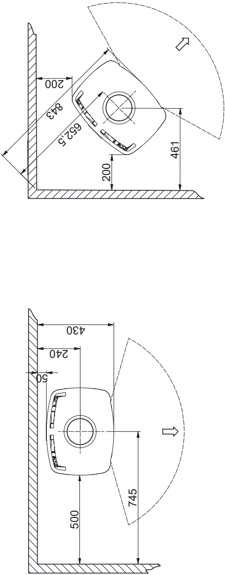
Minimumsavstand til brennbart materiale (uten sideglass)
